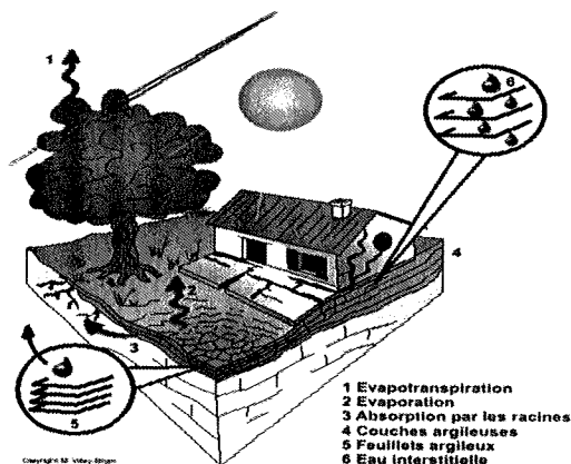
fig. 1 : illustration du mécanisme de dessiccation
