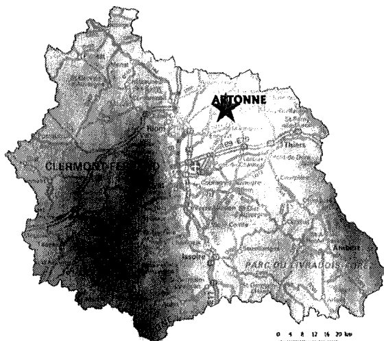
AOT40 en O 3 , en µg.m -1 .h
