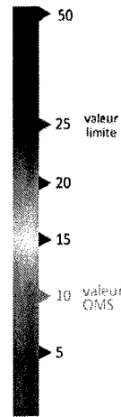
Moyenne annuelle de PM 2.5 en µg.m -3
