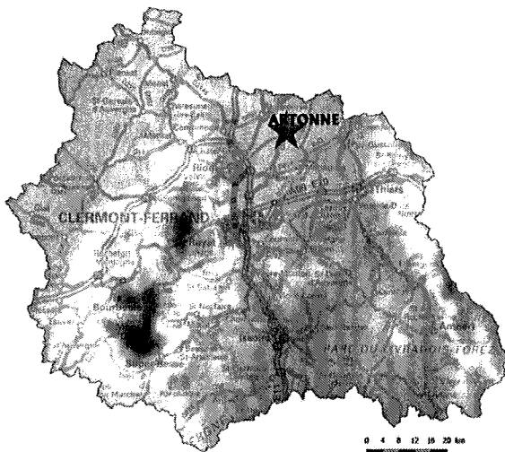
Nombre de jours de dépassement en O 3 (>120µg.m -3 )
