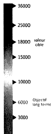
AOT40 en O 3 , en µg.m -1 .h
